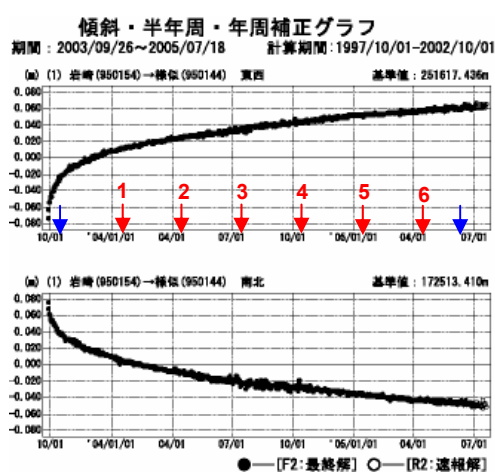
図-10 非正常地殻変動の検出例 (I)
