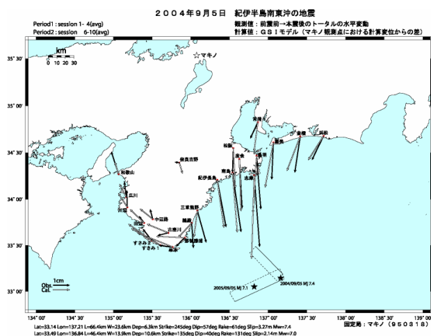
図-12 解析結果(前震前一本震後)と国土地理院(2004)の比較
