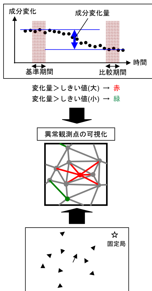
図-1 異常観測点検出の考え方
