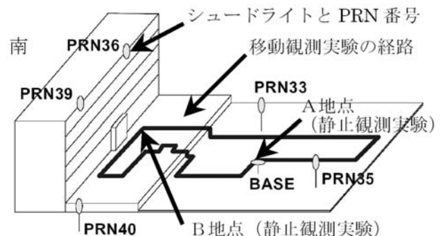
図-5 シュードライトの実験場所と配置図 (小西勇介, 2002に加筆)
