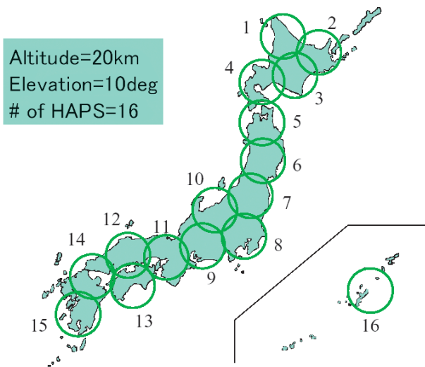
図-4 成層圏プラットフォームの位置例 (三浦龍, 2001)
