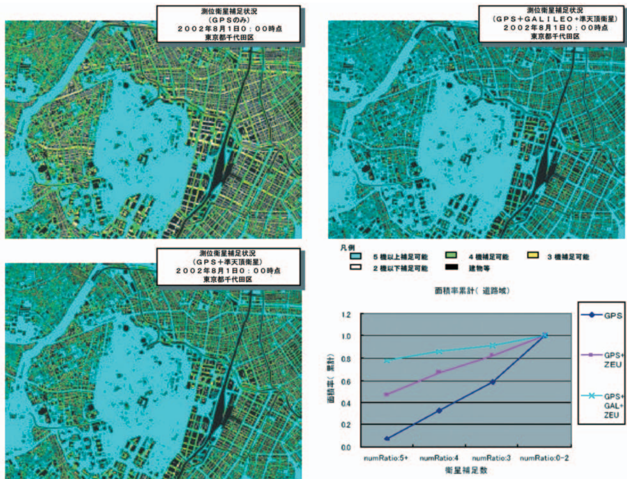
図-2 準天頂衛星の追加による測位可能地域のシミュレーション(総合科学技術会議2002b)
