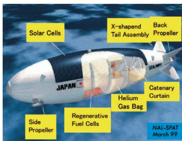
図-3 成層圏プラットフォームの概念図 （航空宇宙技術研究所による）
