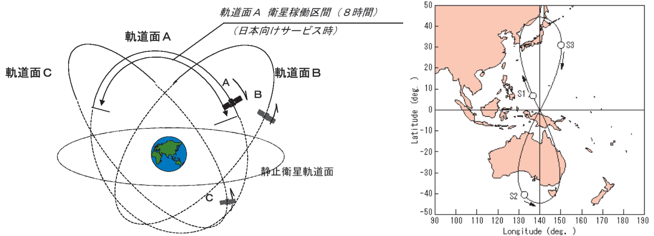
図-1 準天頂衛星の軌道(左)と地上軌跡(右)
