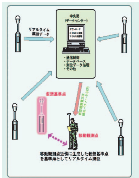
図-28 電子基準点リアルタイムデータを利用した仮想基準点方式のイメージ
