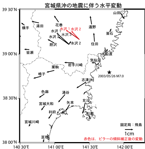
図-31 2003年5月26日に発生した宮城県沖の地震前後の水平地殻変動 基準期間2003/5/16～5/25の平均値に対する5/27～6/5の平均値を示す。赤色のベクトルは、「水沢1」、「水沢2」について地震に伴うピラー傾斜を、傾斜測定結果を元に補正したベクトルを示す。
