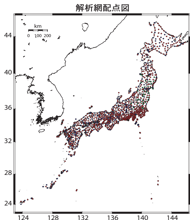
図-30 旧GEONETに存在した3つの解析網 プロットの色で解析網を分類表示している。 赤: Trimble網, 青: Ashtech網, 緑: Leica網
