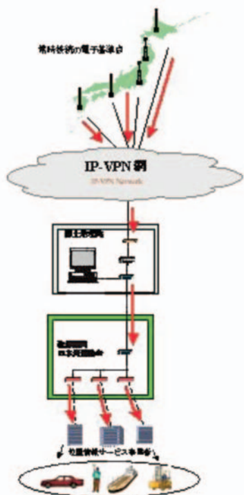
図-27 電子基準点リアルタイムデータの流れ
