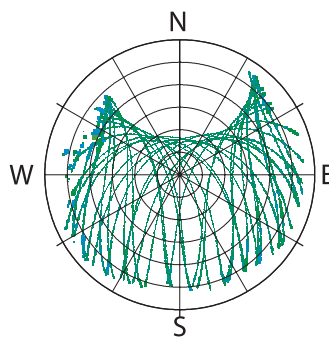
図-32 「館岩」のマルチパスのスカイプロット図
