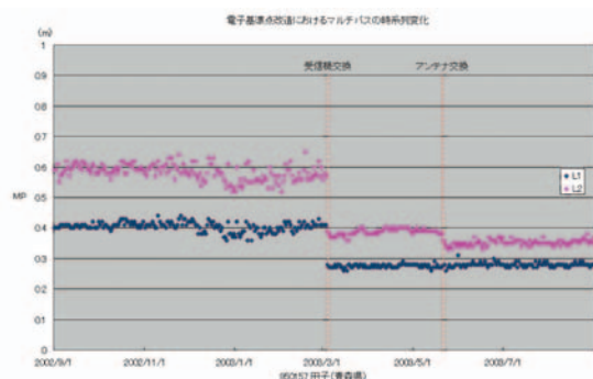
図-29 改造におけるマルチパスの時系列変化
