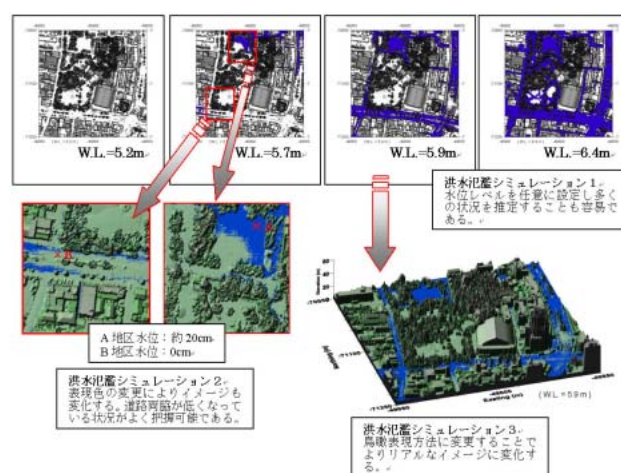
図－18 河川氾濫シミュレーション（大垣市街）
