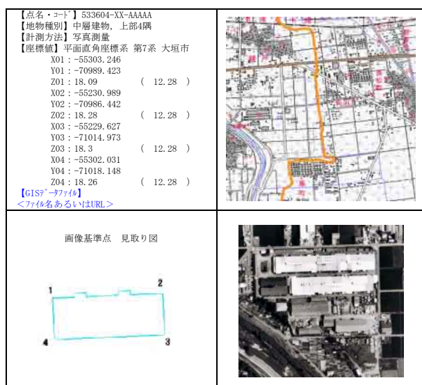
図－20 画像基準点の成果（点の記）
