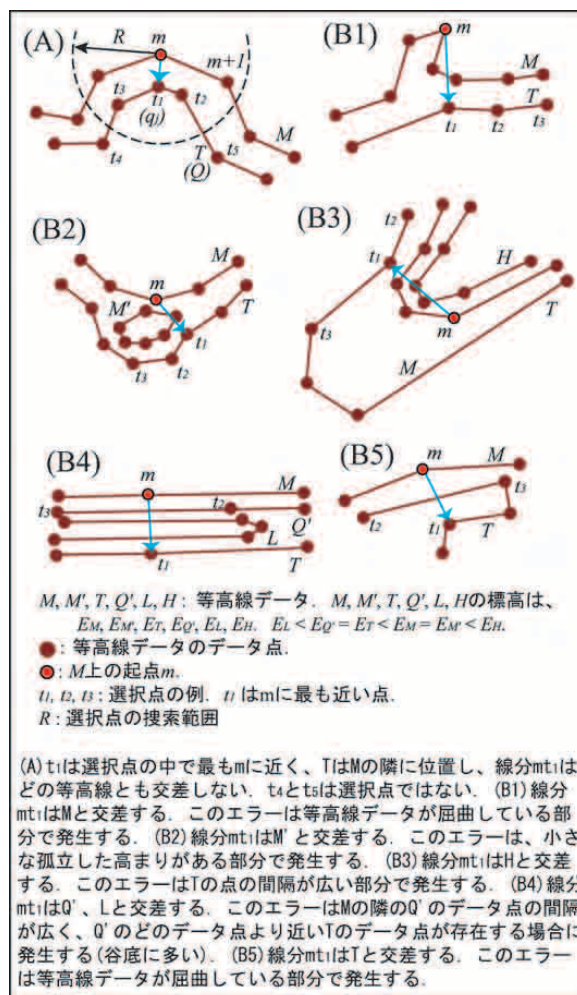
図-3 点 q_j の搜索と決定
