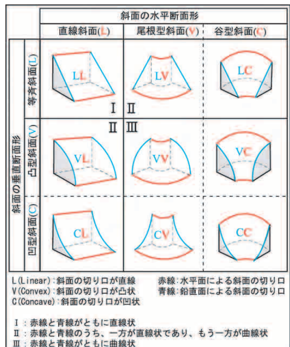
図-1 斜面型の分類 (Dikau (1990) を一部改)
