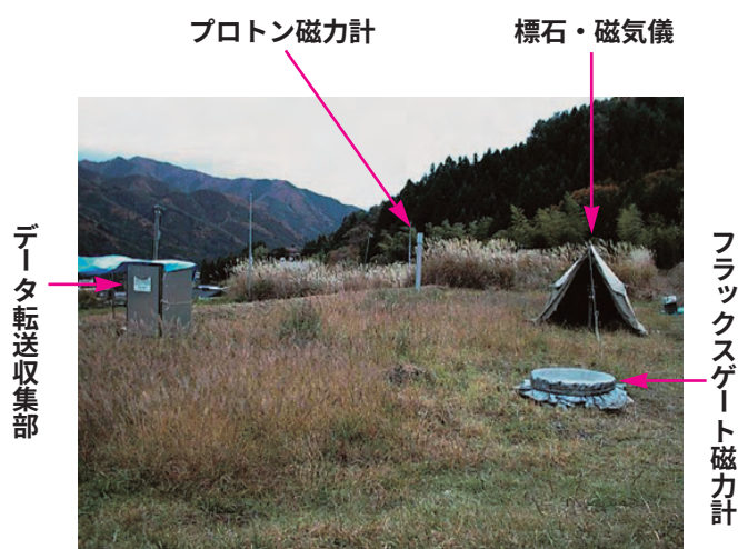
写真－2 地球電磁気連続観測装置の全景 (岐阜県益田郡萩原町)
